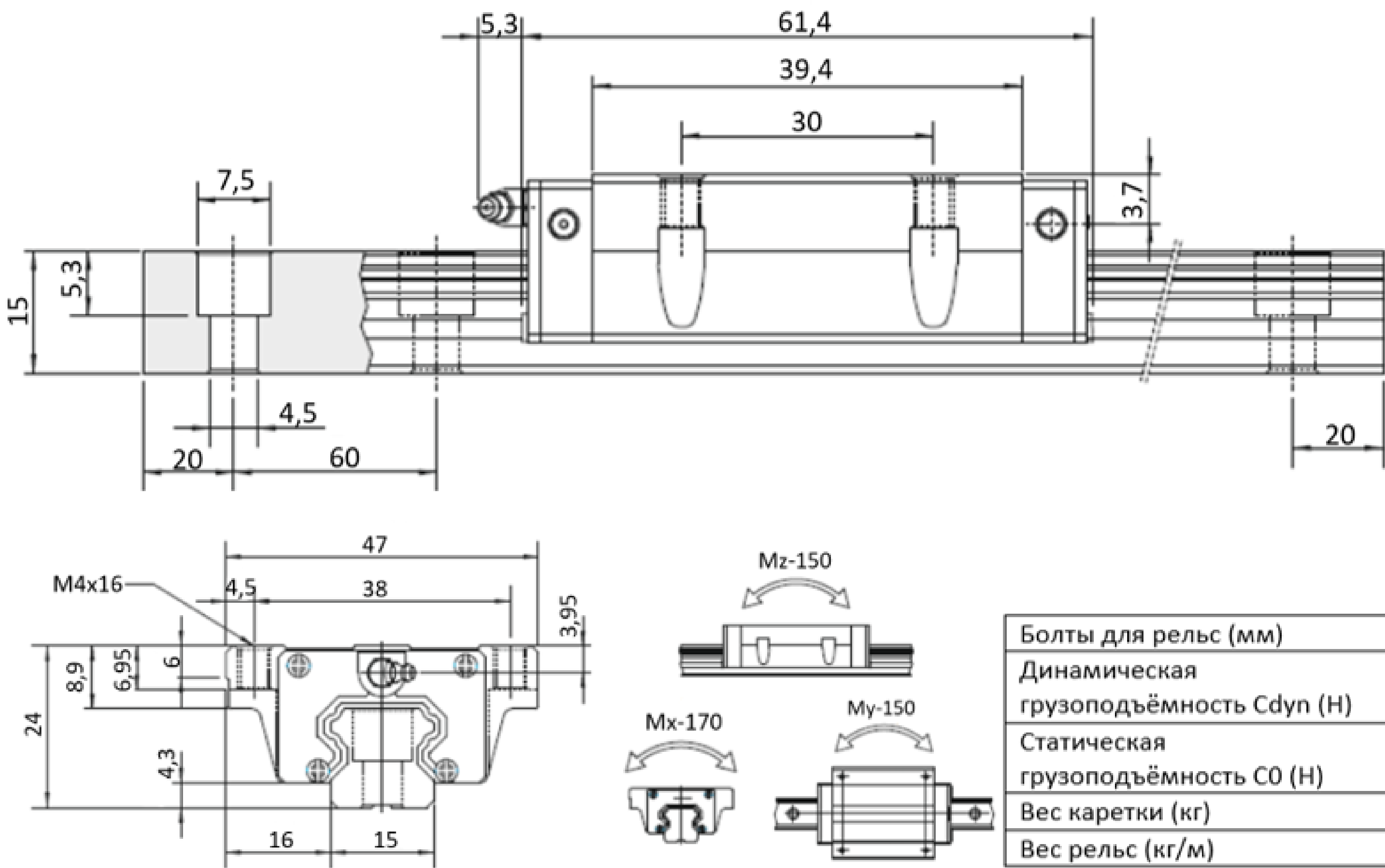
Размеры блока TRH HGW15CA
